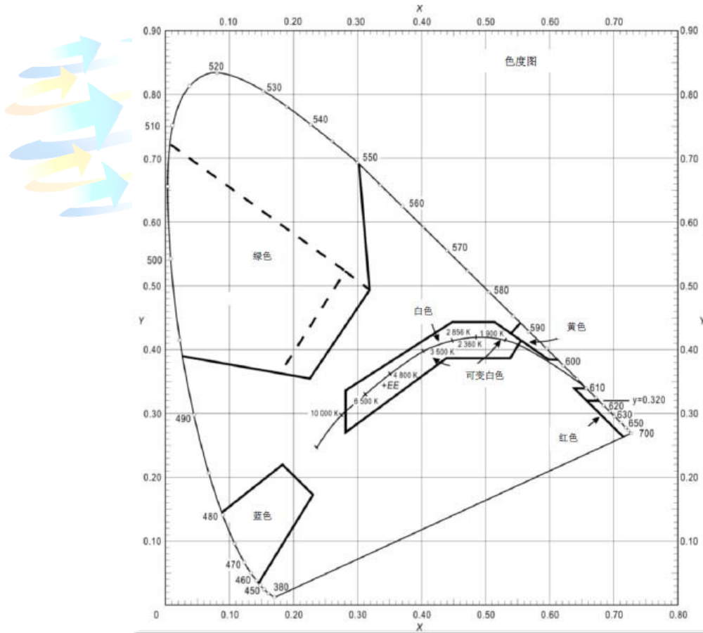
图 1 障碍灯的颜色（气体放电型、电热型光源）
