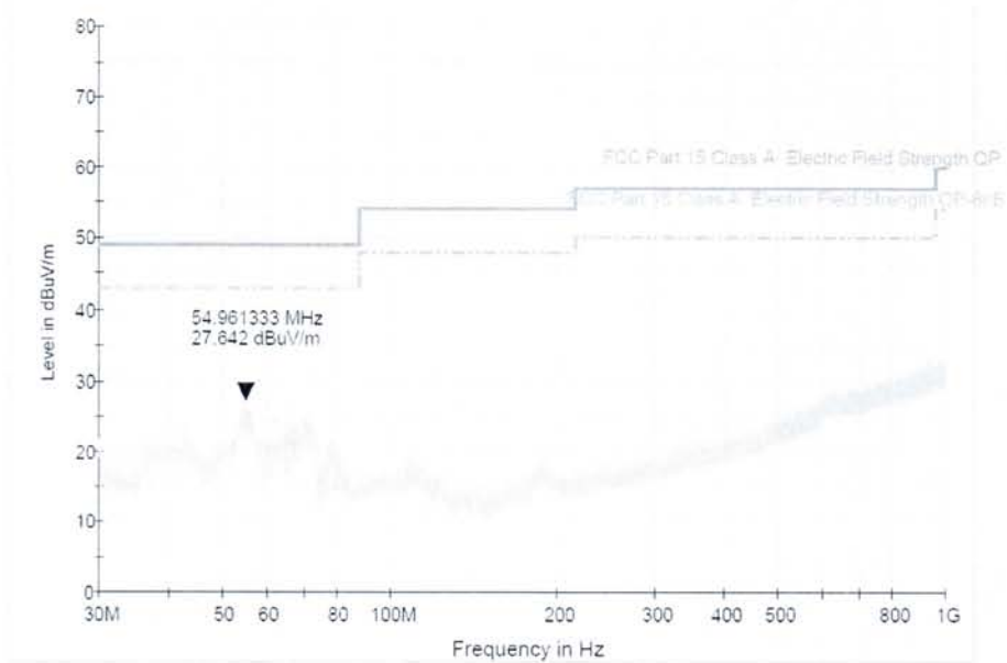
图 9 辐射电磁骚扰 (30MHz~1GHz) 天线水平方向 检测数据
