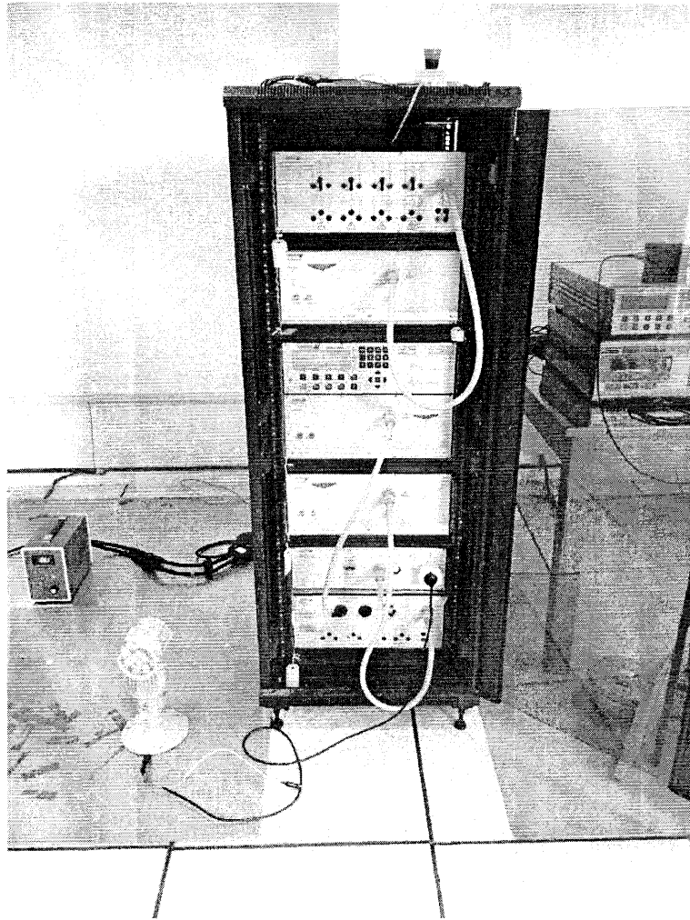
图 16 浪涌抗扰度 被测设备的连接图
