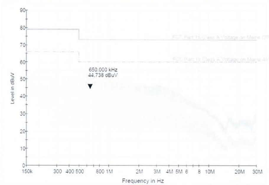
图 8 传导骚扰 (0.15MHz~30MHz) N 相 检测数据
