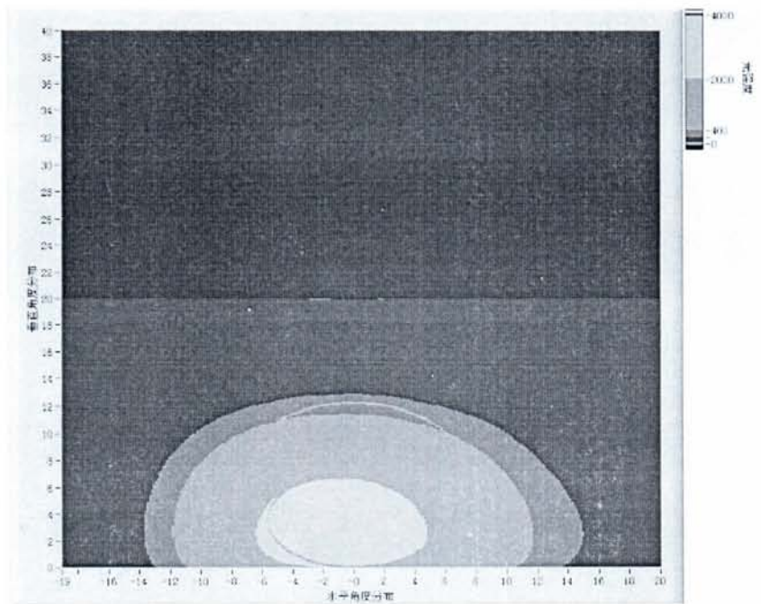
图 6 3#样品发光强度分布（红）
