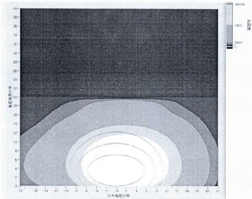
图 1 1#样品发光强度分布（白）
