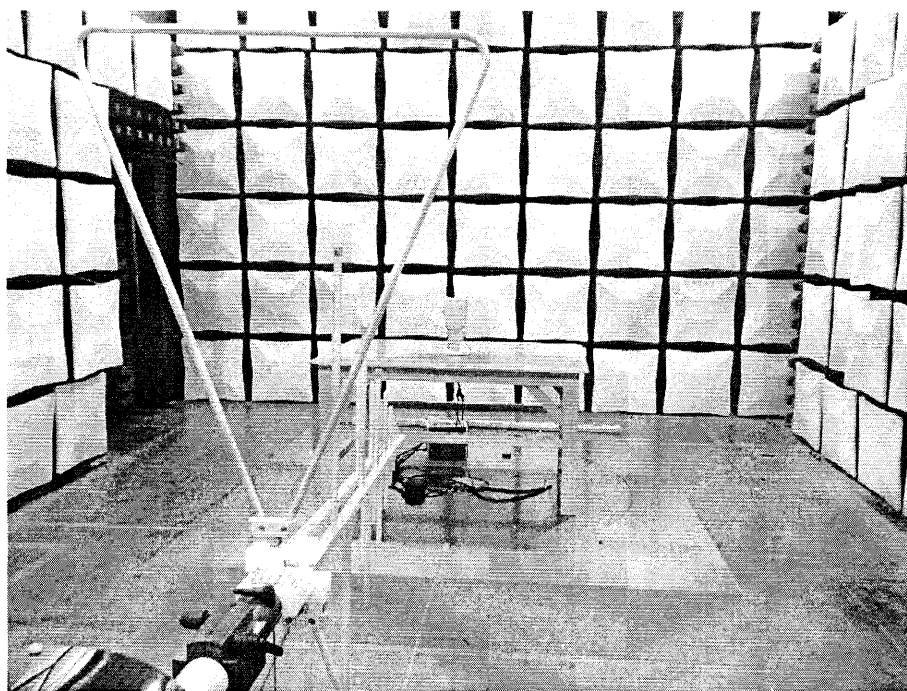
图 15 辐射电磁骚扰 (30MHz~1GHz) 被测设备连接图
