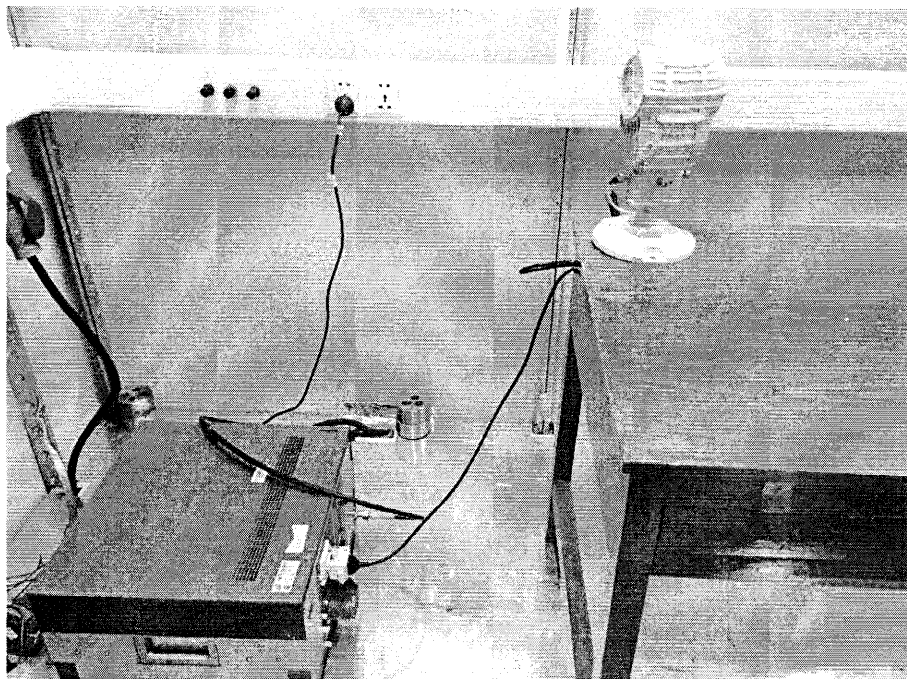
图 14 传导骚扰 (0.15MHz~30MHz) 被测设备连接图
