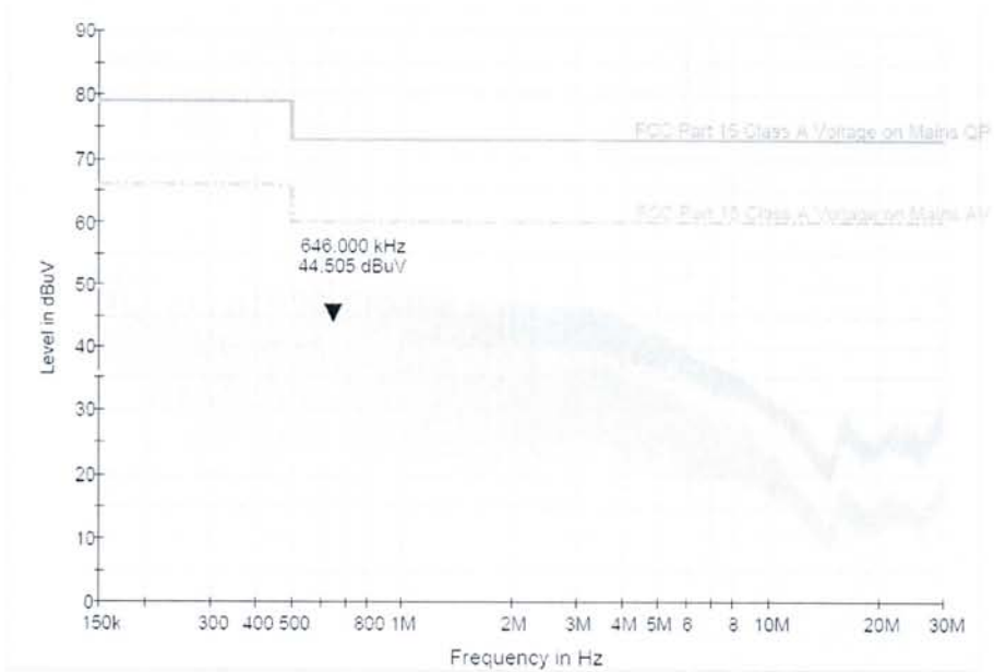
图 7 传导骚扰 (0.15MHz~30MHz) L 相 检测数据
