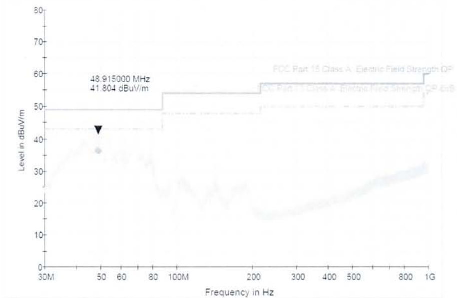
图 9 辐射电磁骚扰 (30MHz~1GHz) 天线水平方向 检测数据
