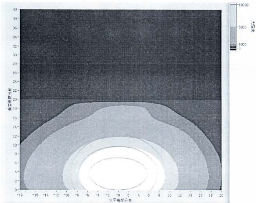
图 5 3#样品发光强度分布（白）
