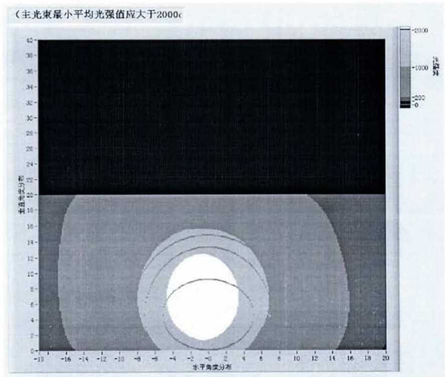
图 1 1#样品发光强度分布
