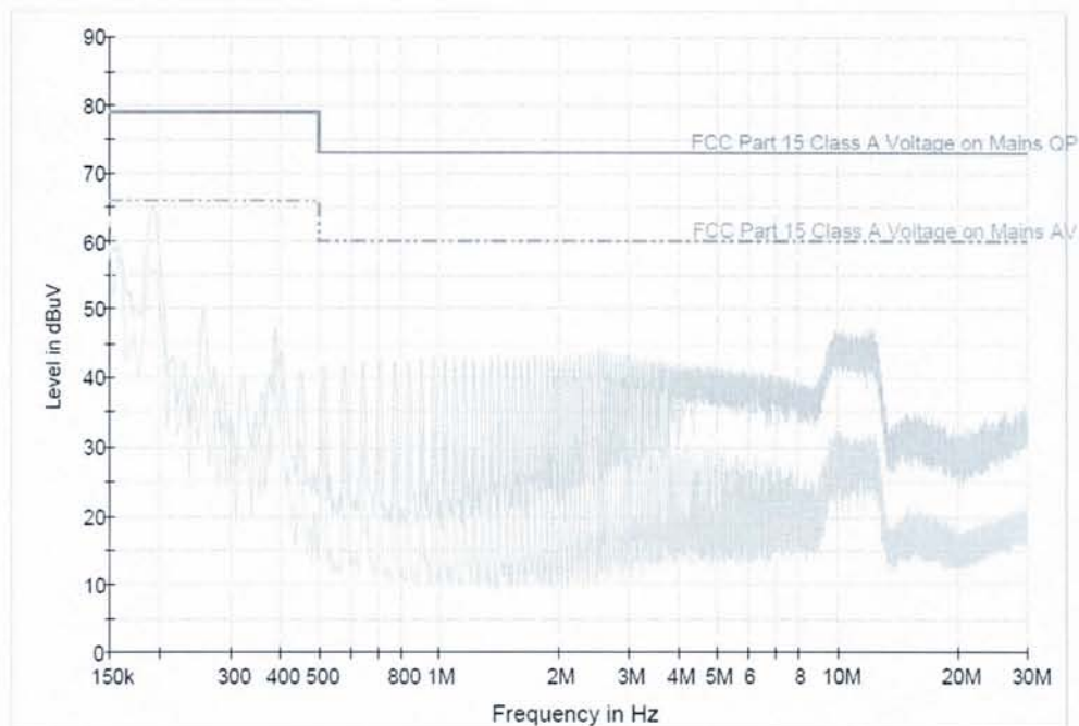
图 4 传导骚扰 (0.15MHz~30MHz) L 相 检测数据
