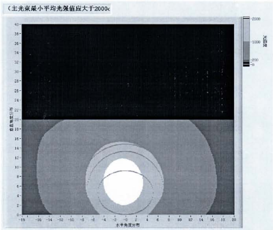
图 3 3#样品发光强度分布
