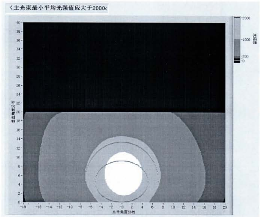
图 2 2#样品发光强度分布
