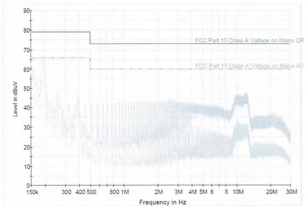
图 5 传导骚扰 (0.15MHz~30MHz) N 相 检测数据
