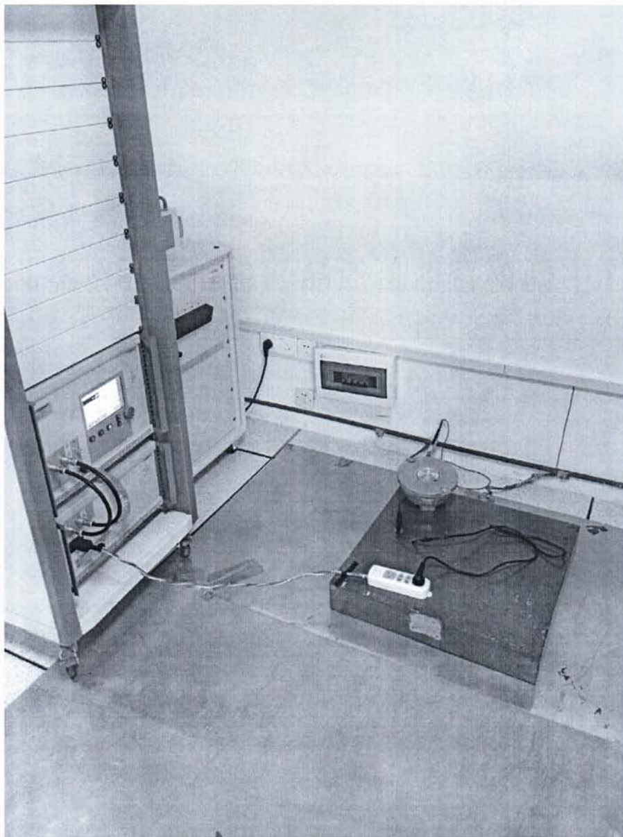
图 10 浪涌抗扰度 被测设备的连接图
