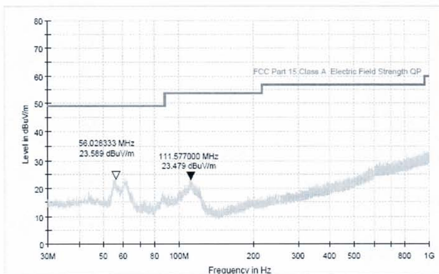
图 4 辐射电磁骚扰 (30MHz~1GHz) 天线水平方向 检测数据
