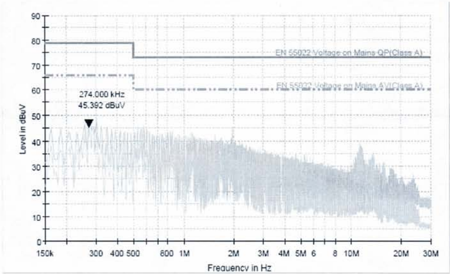
图 1 传导骚扰 (0.15MHz~30MHz) L 相 检测数据
