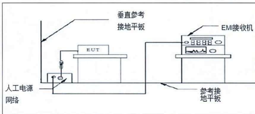
图 5 传导骚扰 检测布置图
