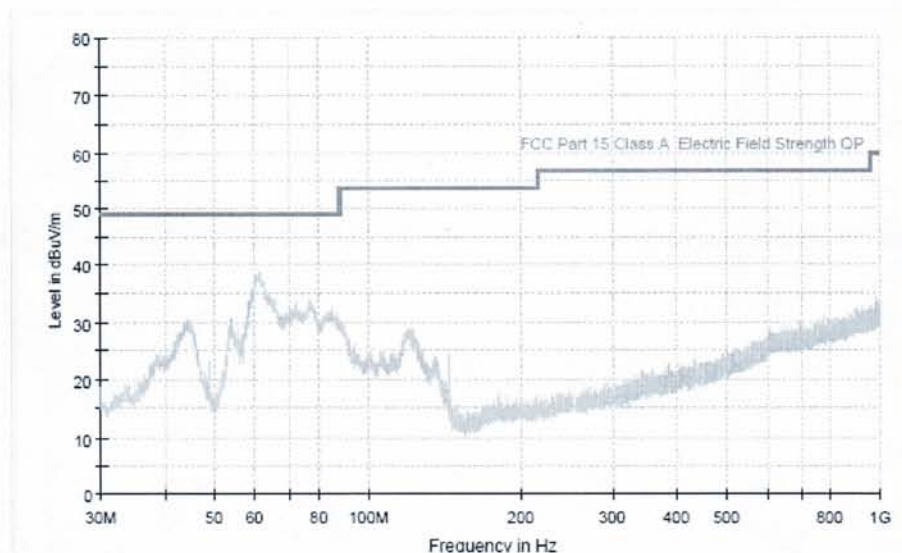
图 3 辐射电磁骚扰 (30MHz~1GHz) 天线垂直方向 检测数据
