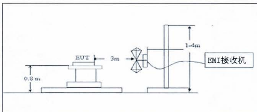
图 6 辐射骚扰 检测布置图
