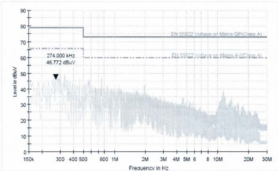
图 2 传导骚扰 (0.15MHz~30MHz) N 相 检测数据
