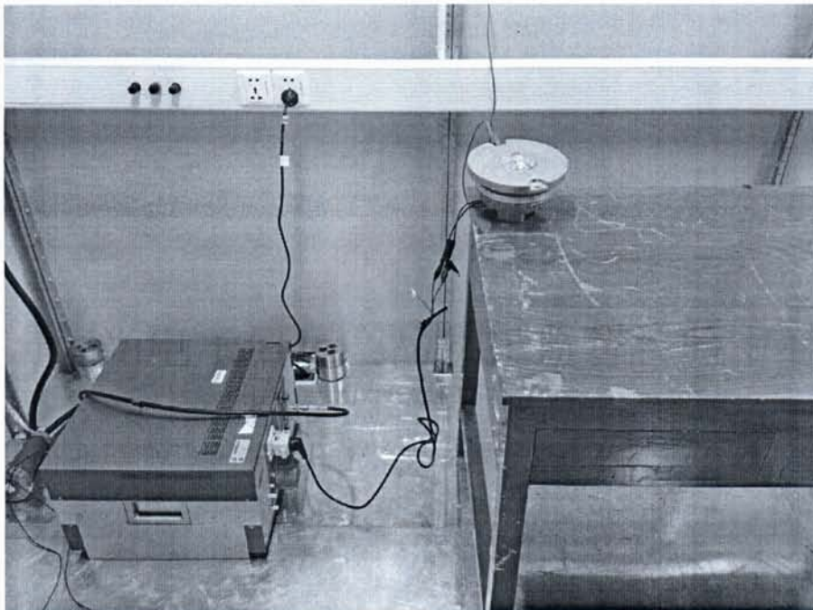
图 8 传导骚扰 (0.15MHz~30MHz) 被测设备连接图
