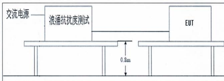
图 7 浪涌抗扰度 检测布置图
