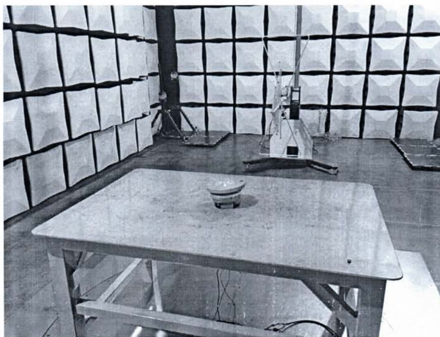
图 9 辐射电磁骚扰 (30MHz~1GHz) 被测设备连接图
